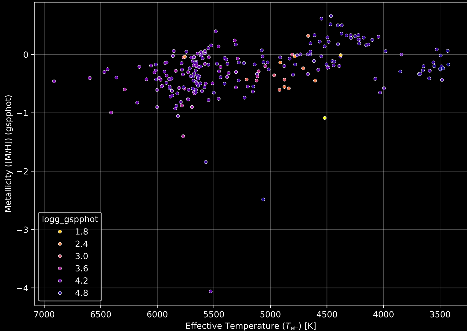
APOGEE DR17 Field: [266+65-O] Stellar Population Parameters (n= 232)
